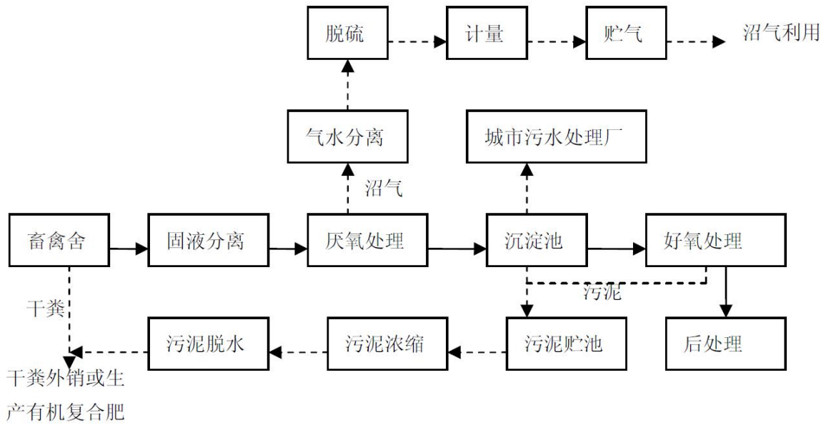
图 4.3-3 厌氧-好氧处理模式工艺流程
